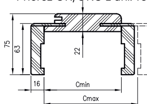
Prierez OR/ORC z uhl. T63
