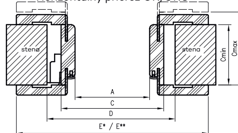
Horizontálny prierez OR/ORC
