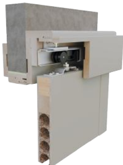
NT systém - inštalovaný pomocou nastaviteľného tunela
