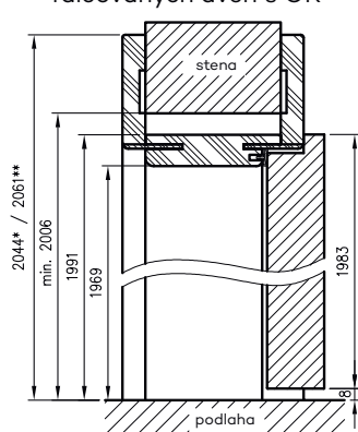
Vertikálny prierez falcovaných dverí s OR
