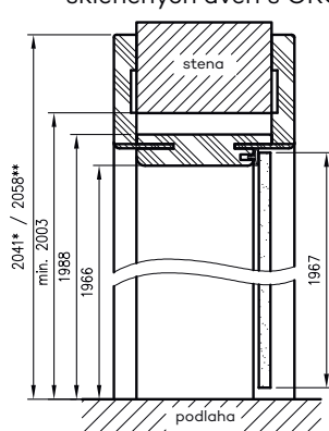
Vertikálny prierez sklenených dverí s ORC
