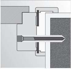
montáž do peny a kotvy do murované steny
