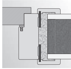
montáž do peny do murované steny
