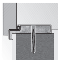
rohová zárubňa veľká montáž pomocou príchytiak
