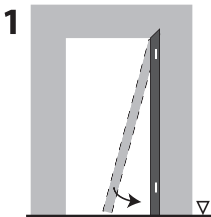
ZVISLÝ NOSNÍK STRANA ZÁVESU
